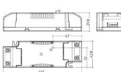
Abmessungen Konverter
