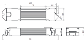
Abmessungen PI-LED LMU
