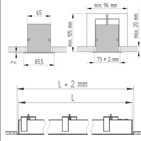
Einbauleuchte recessed luminaire
