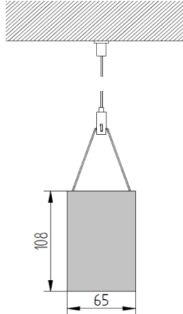
Aufbauleuchte surface-mounted luminaire
